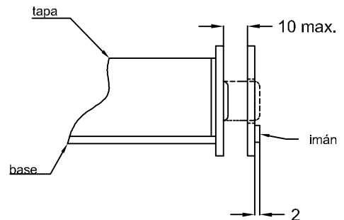
DETALLE PARA LA COLOCACIÓN DEL CERRADERO
