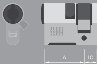
Medio cilindro de perfil tipo BO 02
